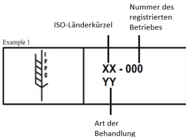
1 Schematische Darstellung eines gültigen ISPM 15 Stempels
